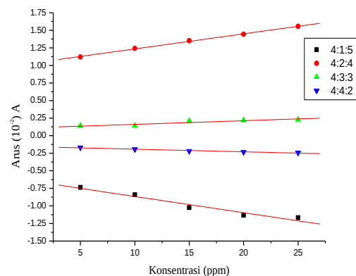
Gbr 6. Kurva EPK Bentonit Berbagai Perbandingan
