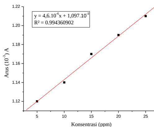
Gbr 9. Kurva Larutan Standar Cu(II)
