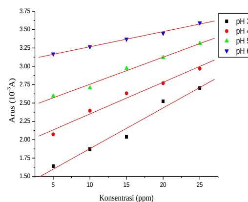
Gbr 7. Kurva EPK Bentonit 4:2:4 dengan Bufer Sitrat
