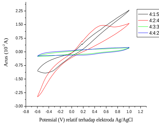
Gbr 4. Grafik EPK Bentonit Teraktivasi
