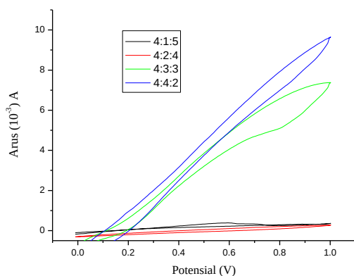
Gbr 3. Grafik EPK Bentonit Nonaktivasi
