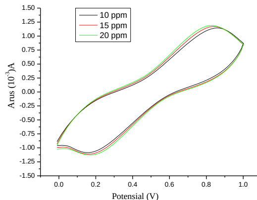
Gbr 8. Voltamogram pengukuran Cu(II) 10 ppm, 15 ppm dan 20 ppm pada pH 6 dengan EPK bentonit 4:2:4
