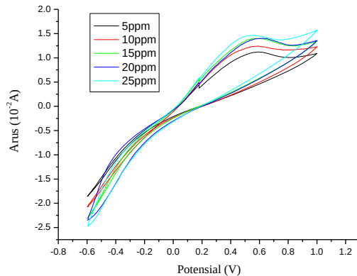
Gbr 5. Voltamogram Cu(II) dengan perbandingan EPK Bentonit 4:2:4
